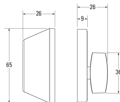
DIMENSIONES (mm)
